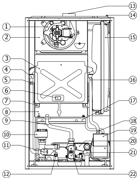
Рисунок 25. Компоненты котла
