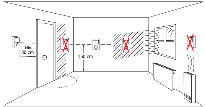
Рисунок 31. Положение термостата
