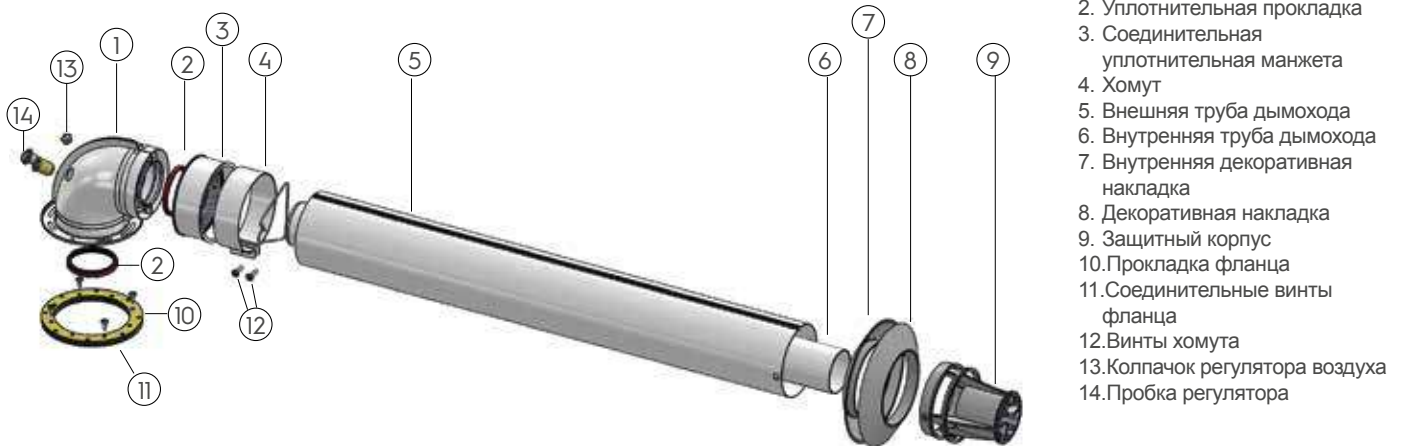
Рисунок 11. Дымоход котла
